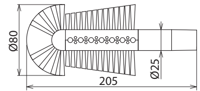
Maßbild STB 80 K MS
