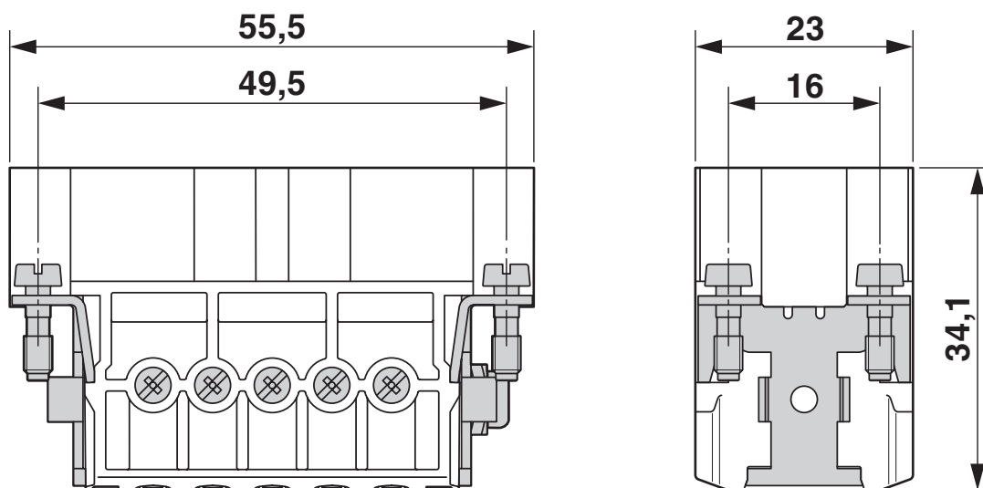
Dessin coté
