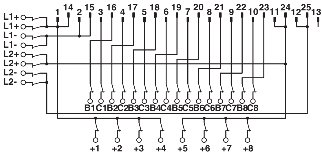
Esquema de conexiones FLKM-D25 SUB/B/KDS3-MT/TU810/P
