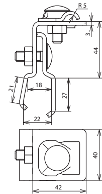
Maßbild DLH KB 6.10 KF18.22 AL
