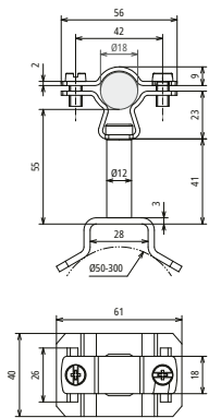
Maßbild LH ZS 18 EX P55 SBB V2A
