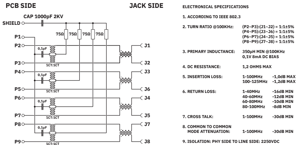
Diagrama eléctrico
