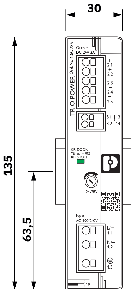
Dessin coté
