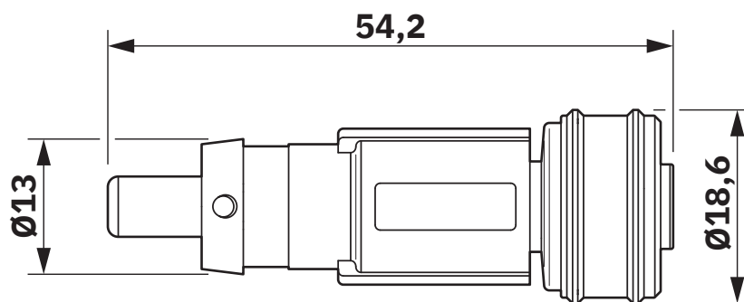
Maßzeichnung
