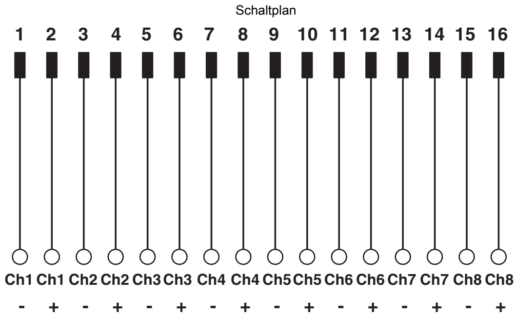
Anschlussbild FLKM 16/DV
