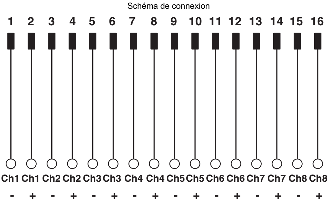
Schéma des connexions FLKM 16/DV
