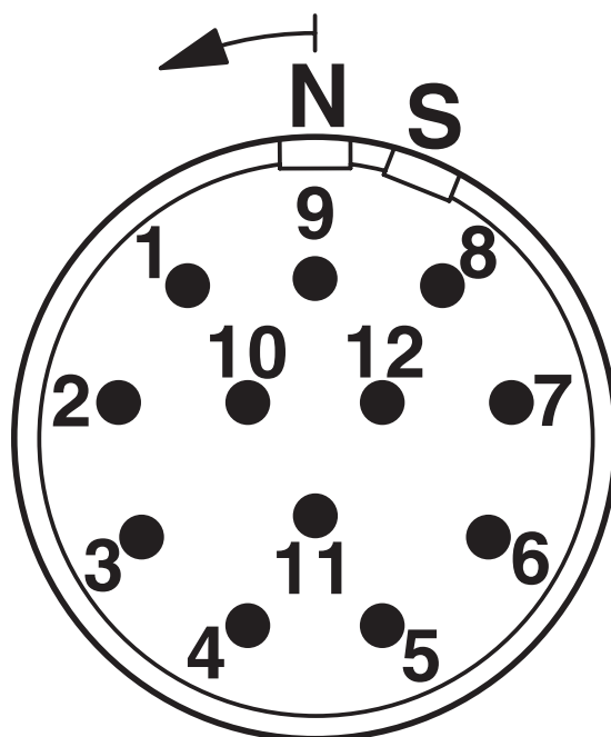
Schemazeichnung
