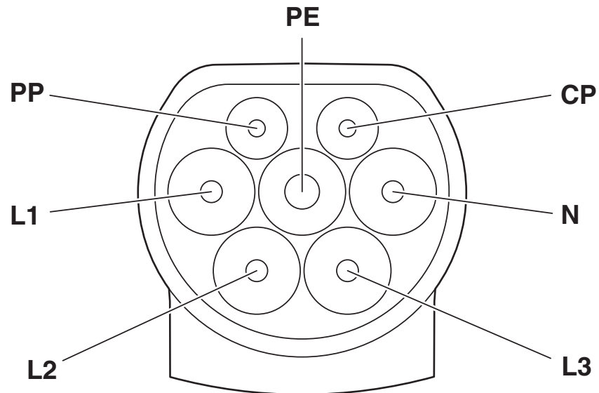
Anschlusszeichnung
