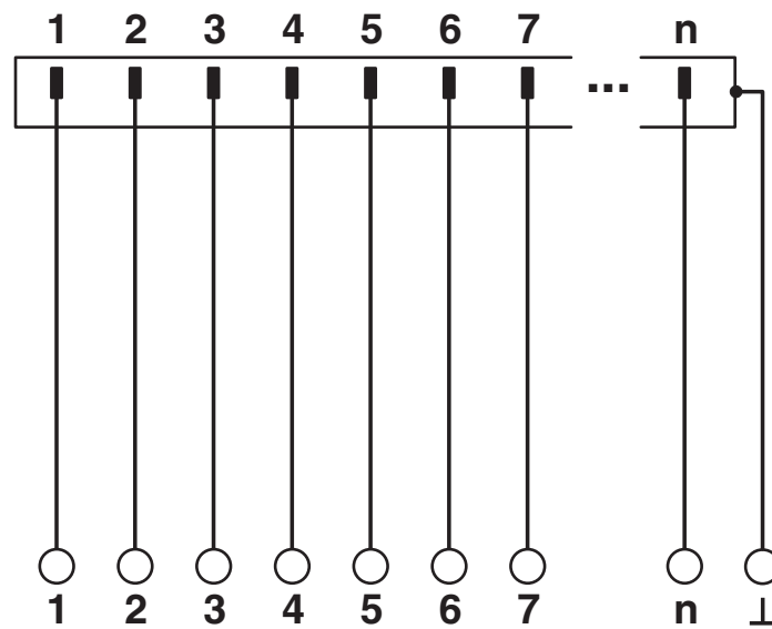
Diagrama eléctrico
