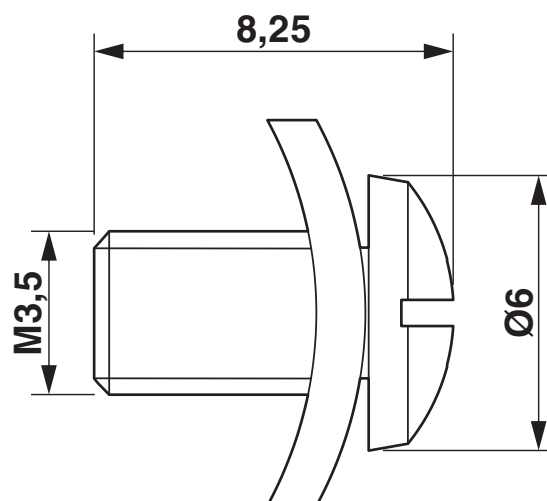
Dessin coté
