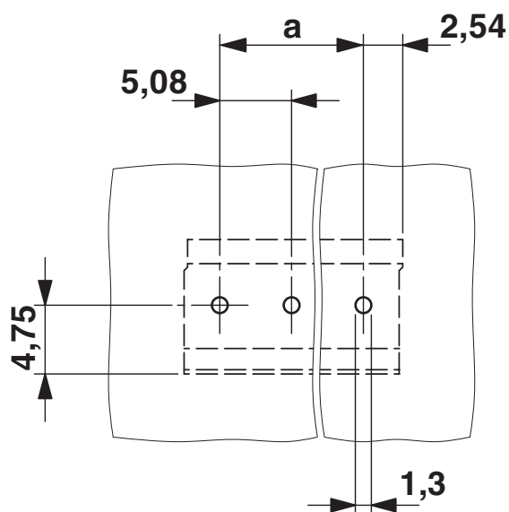
Bohrplan/Lötpadgeometrie
