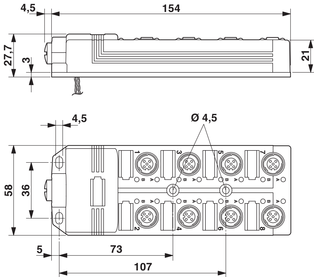
Dessin coté
