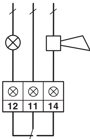
Schéma de l'application schématique
