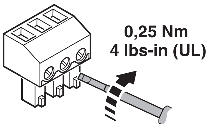
Dessin schématique
