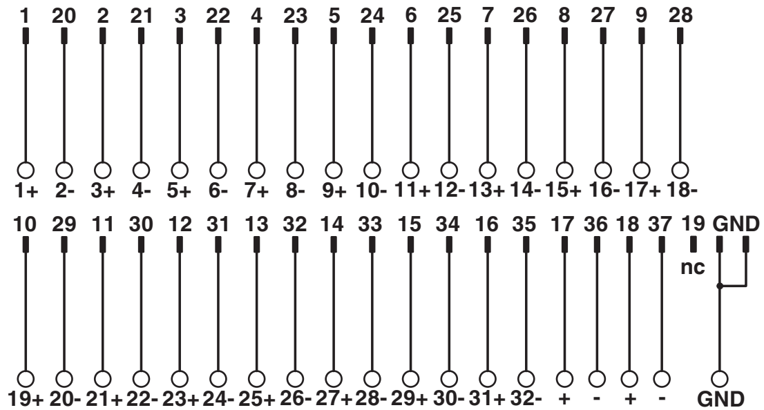
Anschlussbild VIP-2/.../D37SUB/M/SO
