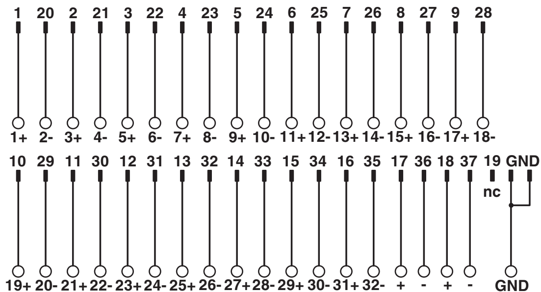
Schéma des connexions VIP-2/.../D37SUB/M/SO
