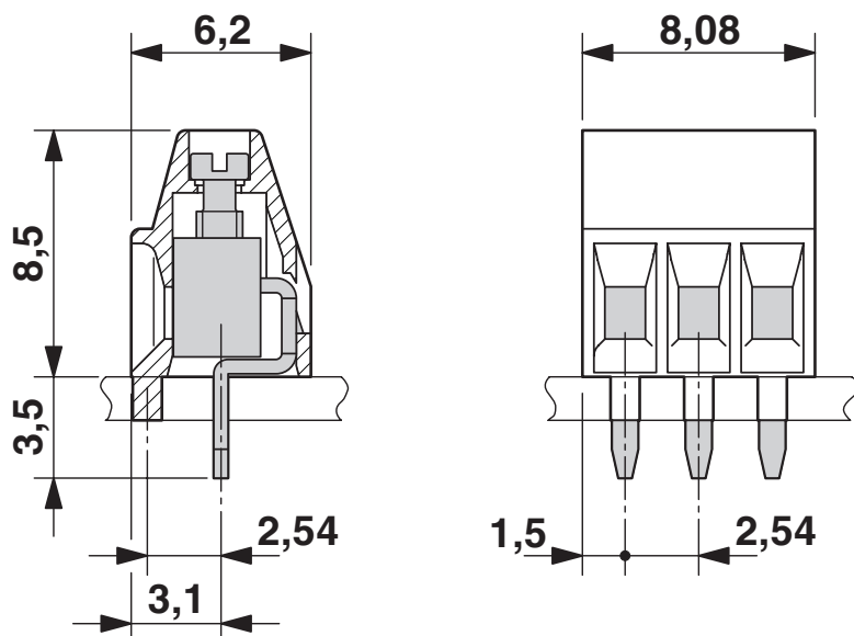
Maßzeichnung
