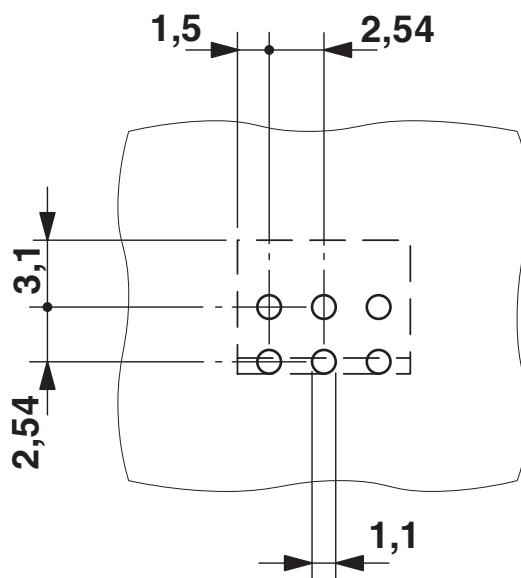
Bohrplan/Lötpadgeometrie
