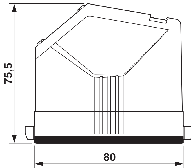
Maßzeichnung
