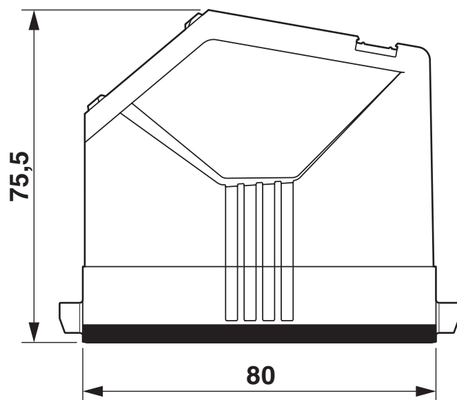
Dessin coté
