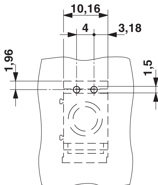
Bohrplan/Lötpadgeometrie
