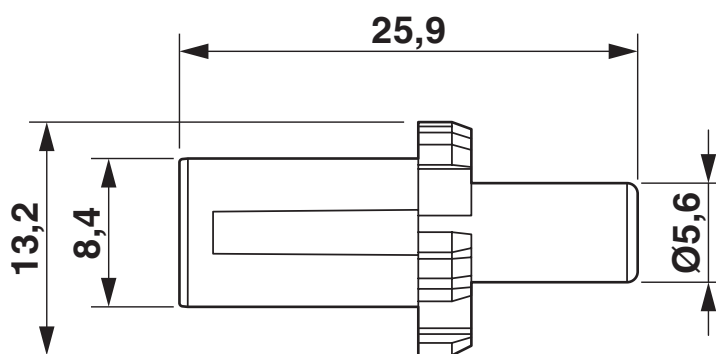
Maßzeichnung
