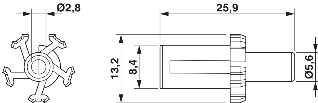
Dessin coté
