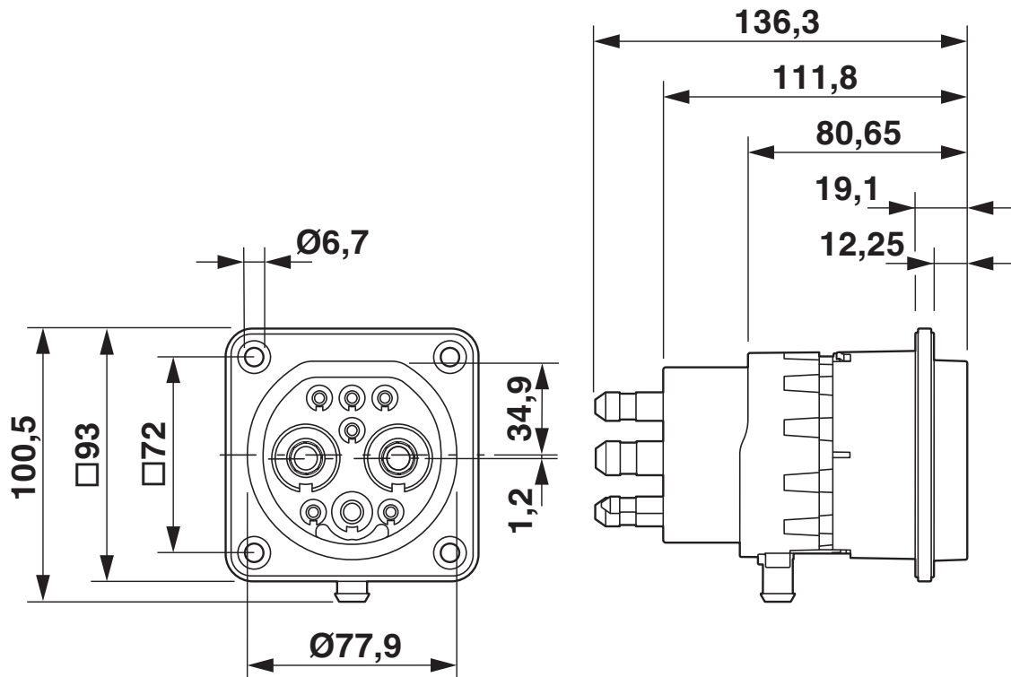
Dessin coté
