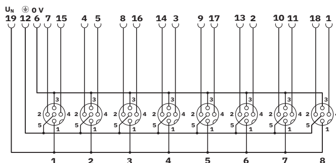
Diagrama eléctrico
