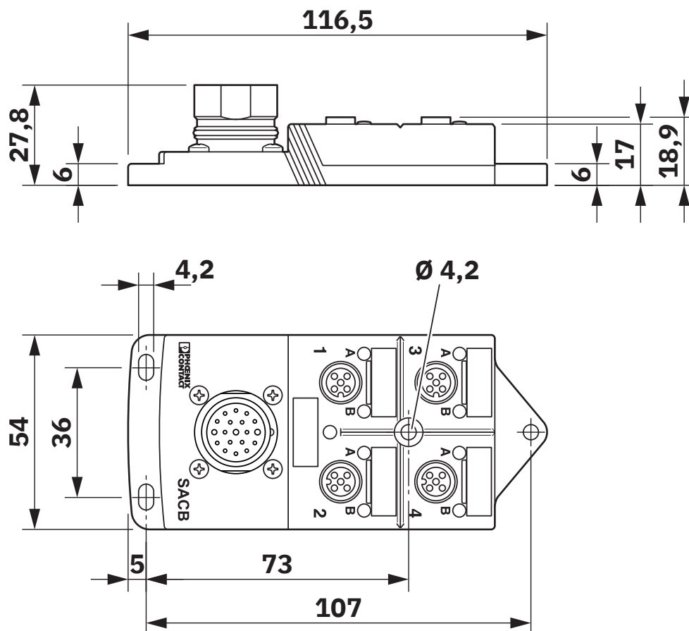
Dessin coté
