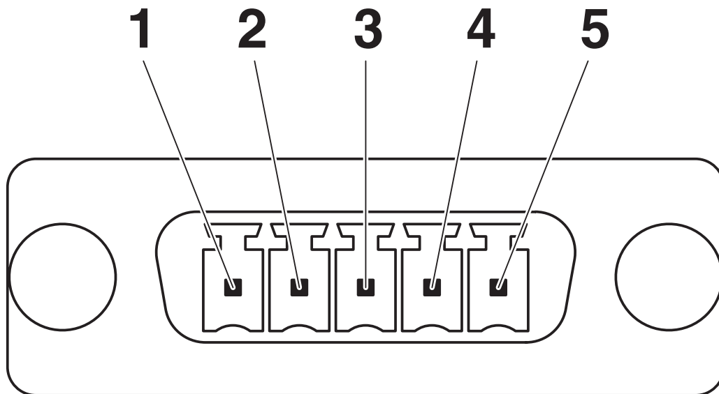
Schemazeichnung
