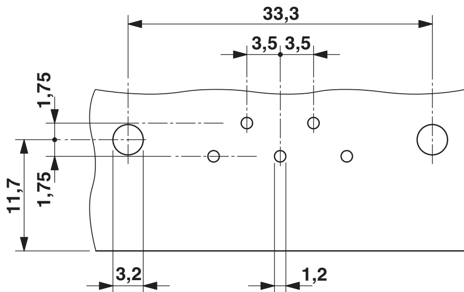
Bohrplan/Lötpadgeometrie
