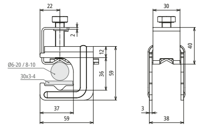
Maßbild VK DB KR 6.20 8.10 FL30 BSB STBL
