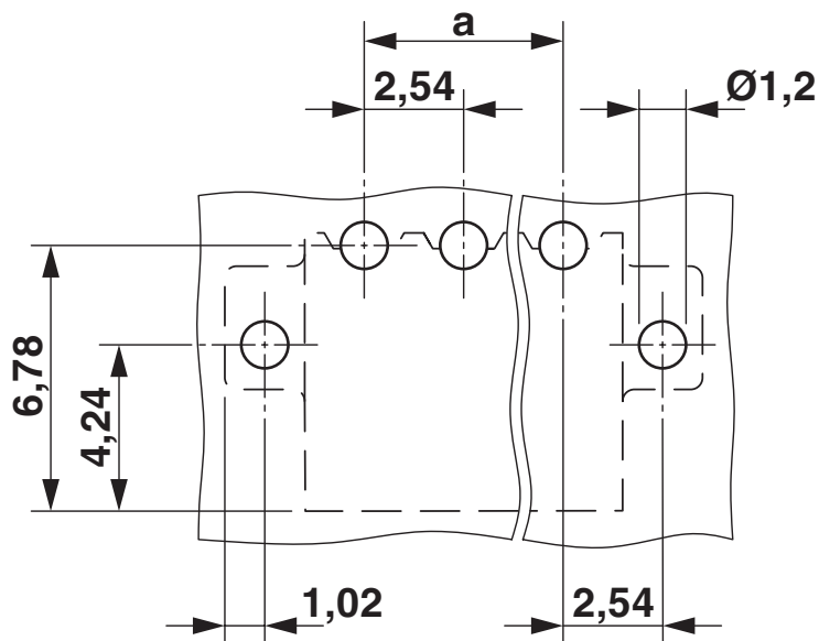
Bohrplan/Lötpadgeometrie
