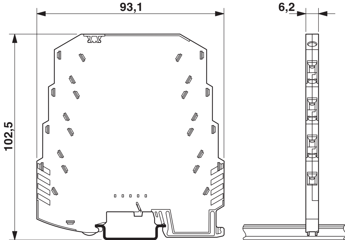
Maßzeichnung
