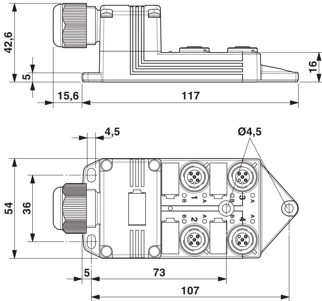
Dessin coté
