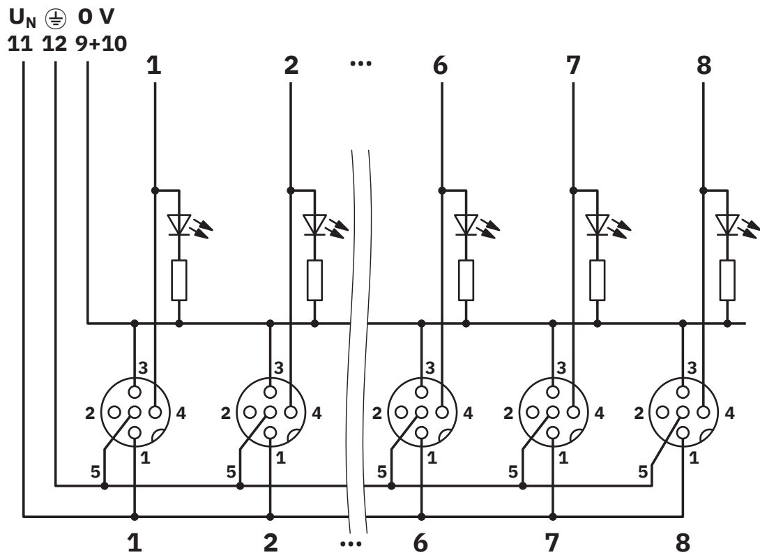
Diagrama eléctrico
