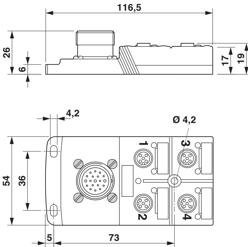
Dessin coté
