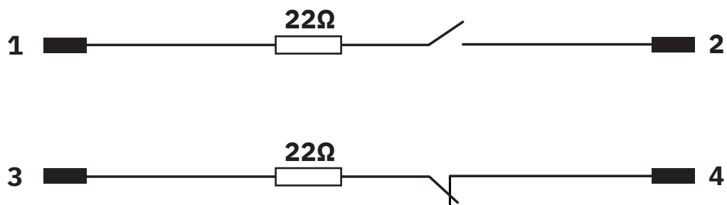
Diagrama eléctrico
