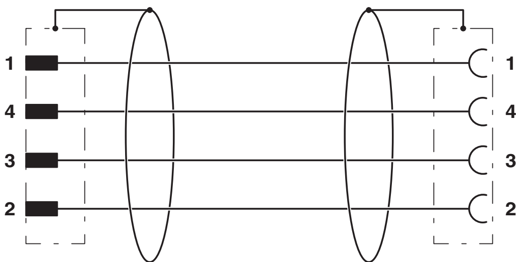
Kontaktbelegung der M12-Stecker / M8-Buchse
