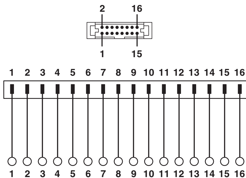
Diagrama eléctrico
