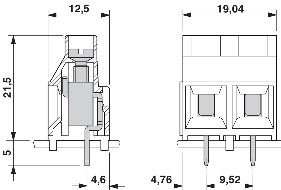
Dessin coté
