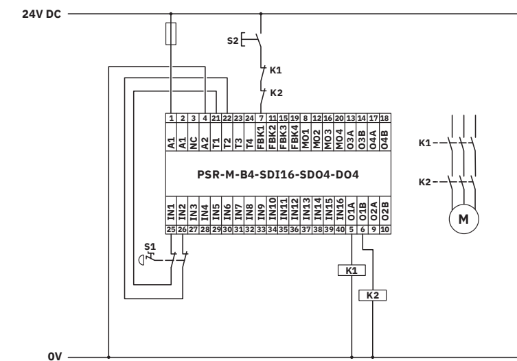
Diagrama eléctrico
