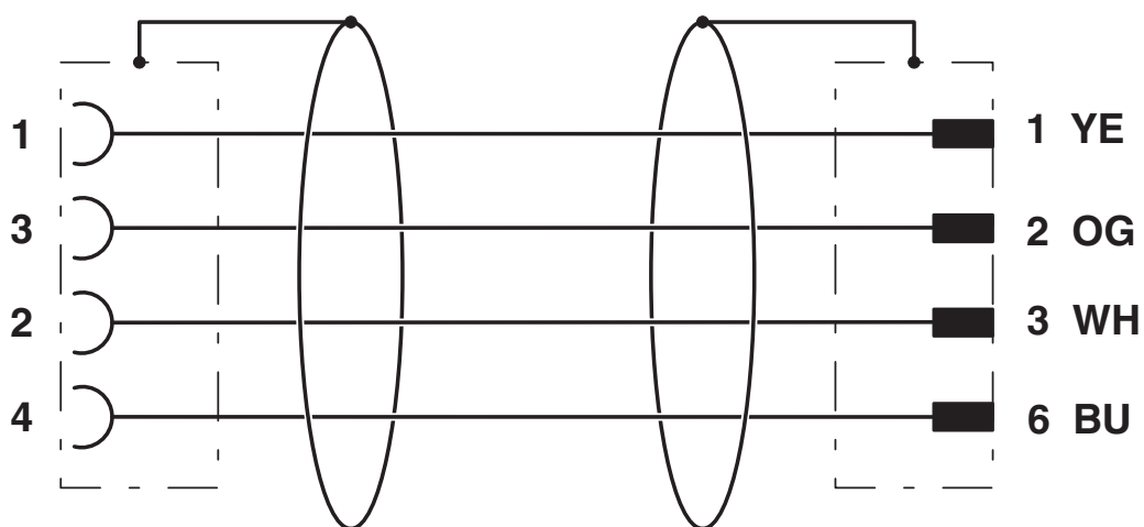
Diagrama eléctrico
