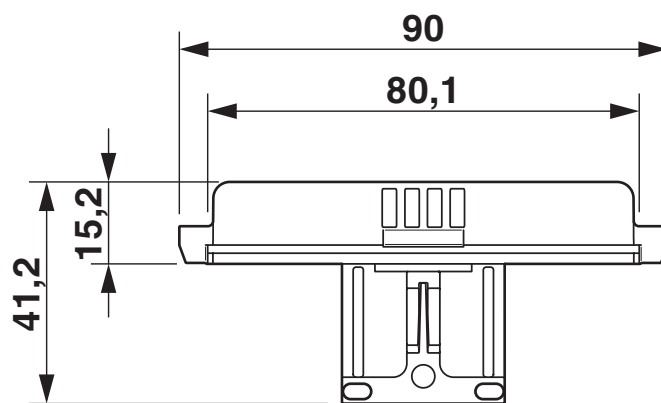
Dessin coté
