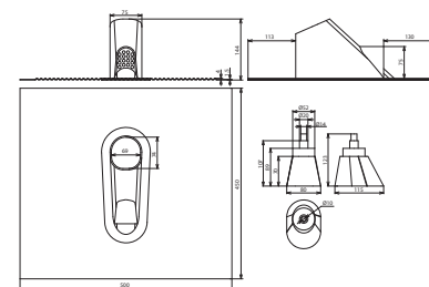
Maßbild DADS D10 16 48 AL ROT
