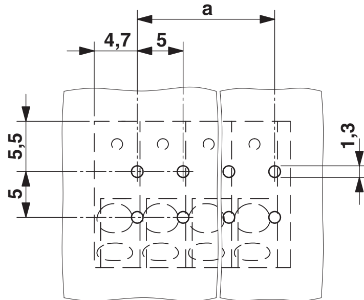
Bohrplan/Lötpadgeometrie
