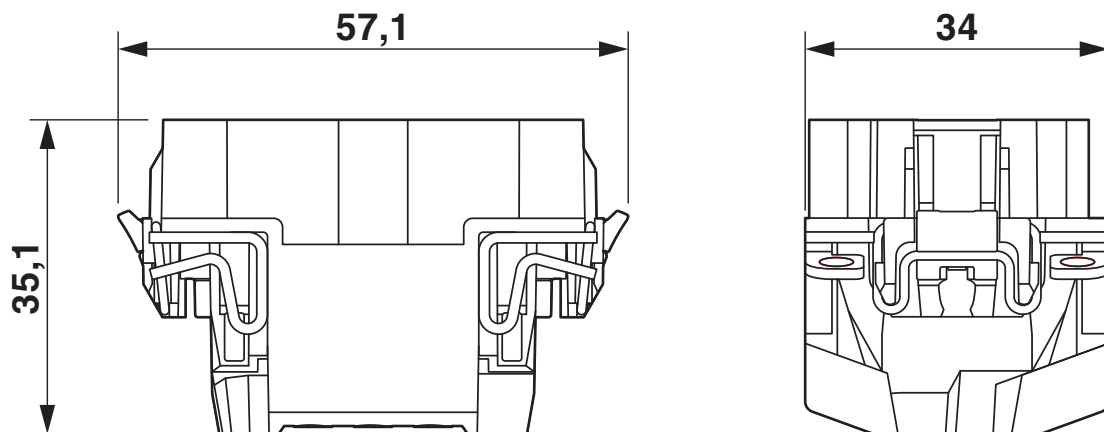
Maßzeichnung
