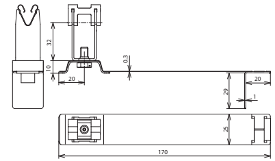
Maßbild DLH FG 8 H32 L170 V2A GALCU
