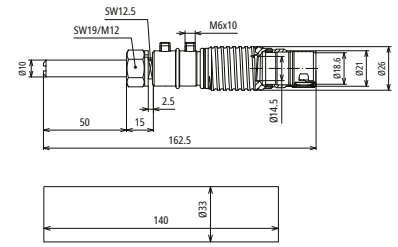
Maßbild AE ISO BO10 KF HVI 60 V2A
