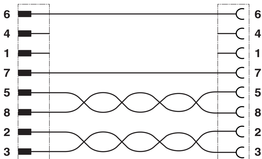
Diagrama eléctrico
