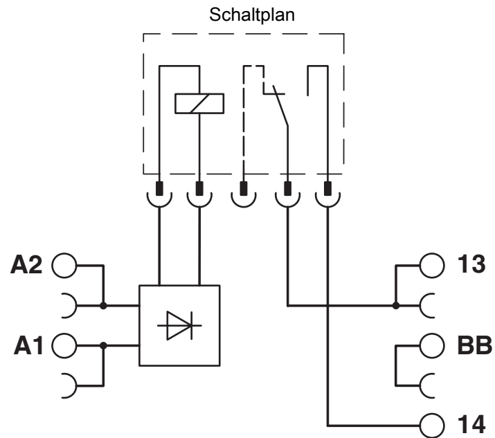
Schaltplan
