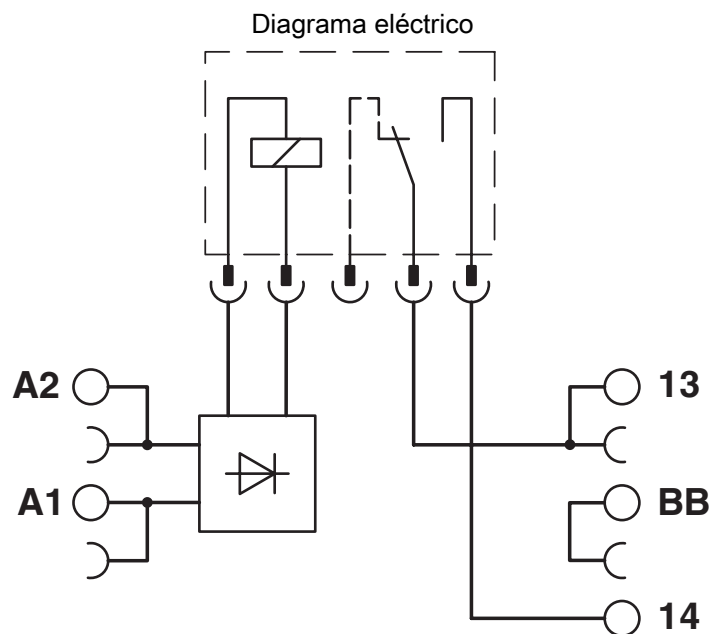
Diagrama eléctrico
